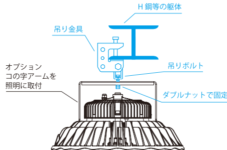
オプションコノ字アームで天井設置
