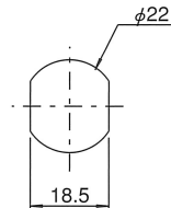
パネル穴明寸法 S=1/1
