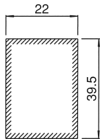
パネル穴明寸法
