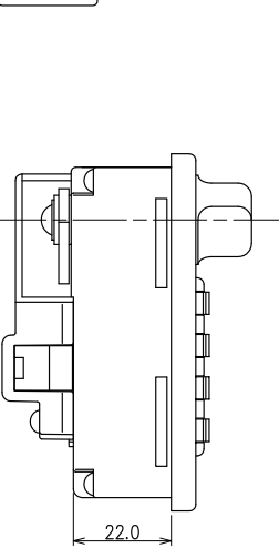
左側面図
