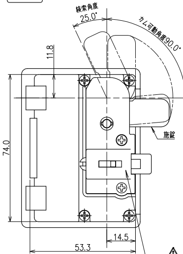
背面図
