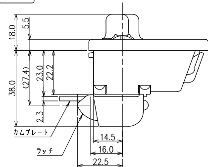
下面図
