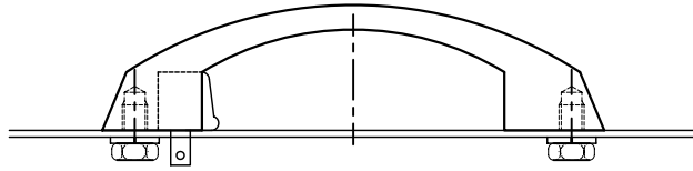
●引手装着図
